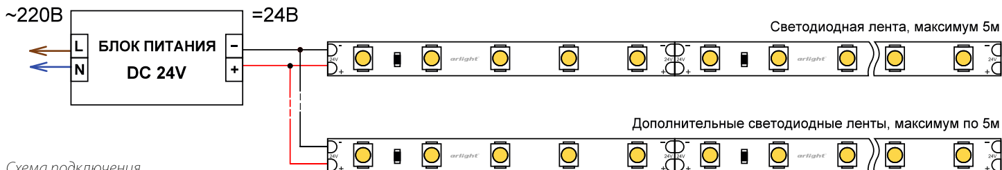
Схема подключения
